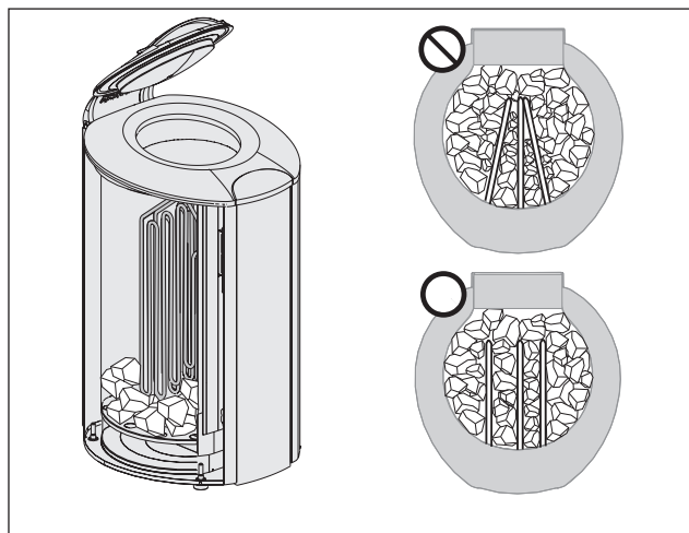
Рис. 5. Положение нагревательных элементов. Joonis 5. Kütteekehade toestamine.
