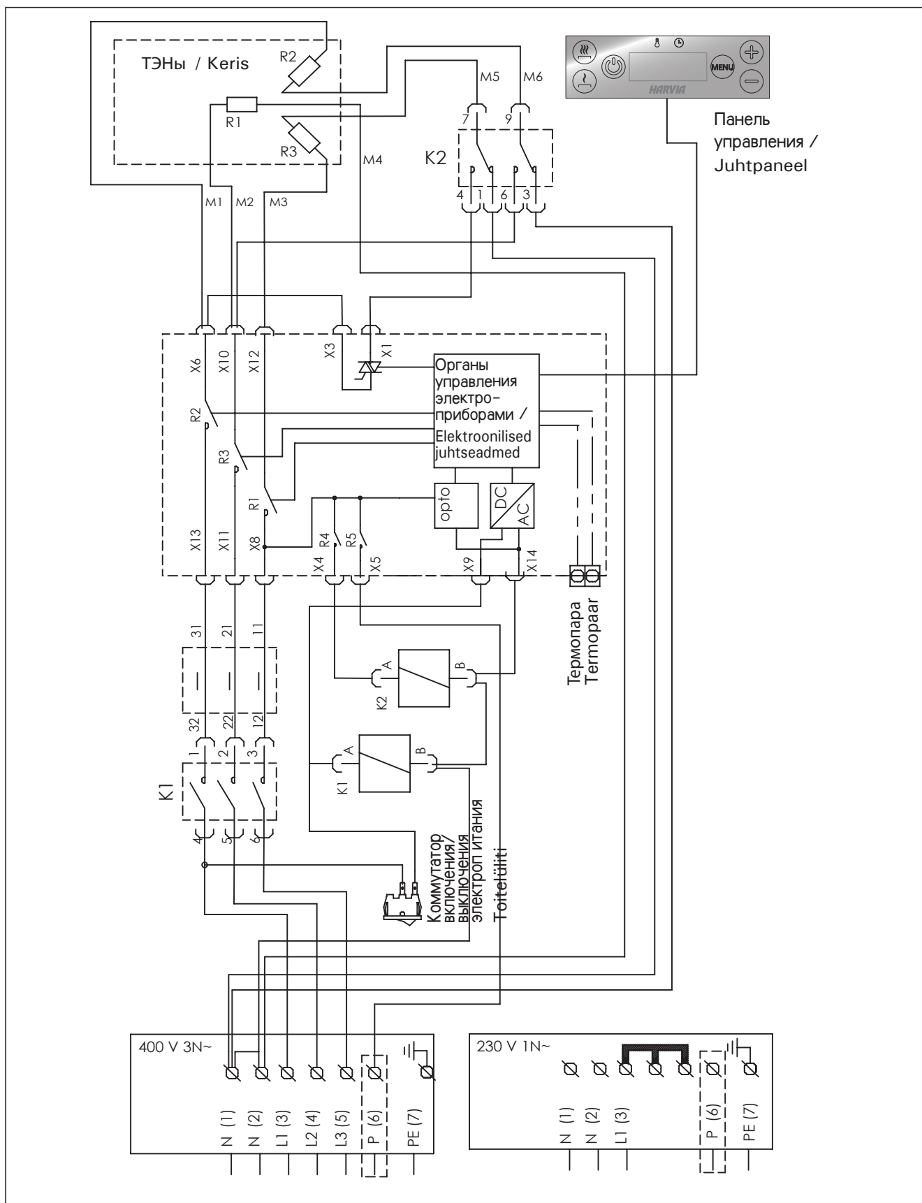
Рис. 12. Электромонтаж каменки Joonis 12. Kerise elektrilised ühendusskeemid
