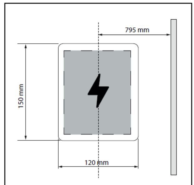
Fig. 2 Mått för montering, vatten- och elanslutning
