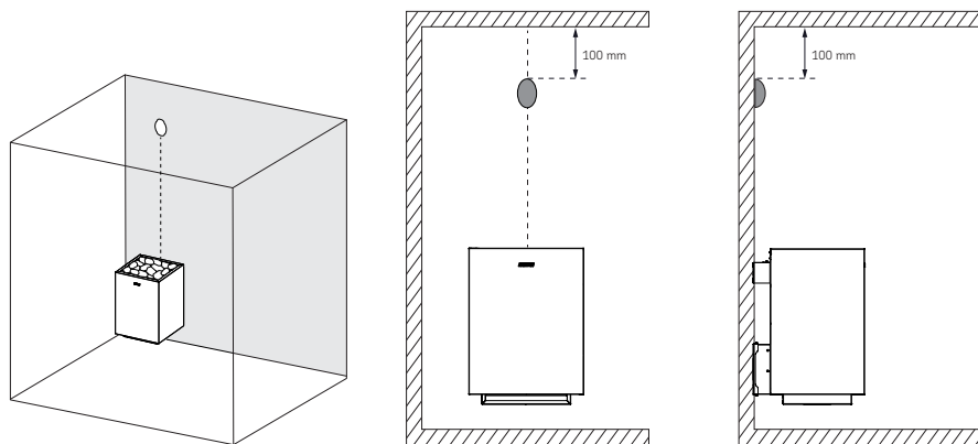
Obrázek 3. Instalace tepelného senzoru na stěnu
