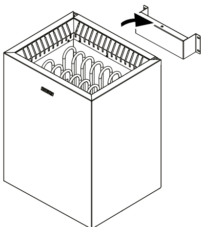
Bild 2. Installation av bastuaggregat
