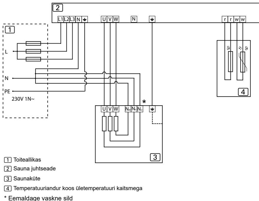
Joonis 10. Elektriskeem 230V 1N~
