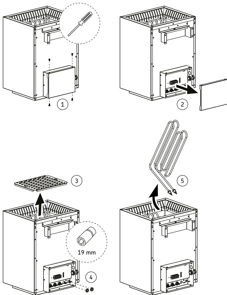
14 pav. Kaitintuvų keitimas
