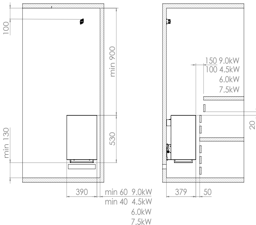
Kuva 1. Suojaetäisyydet
