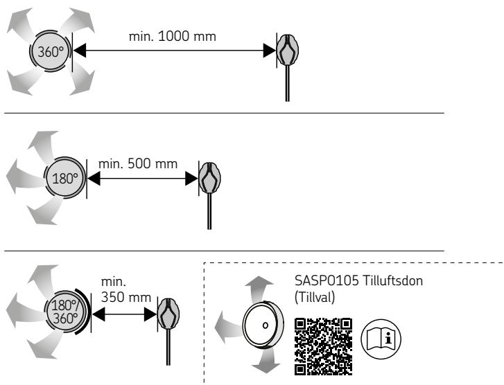
Bild 13. Minimiavstånd mellan tilluftsventil och temperaturgivare.
