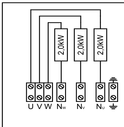
Rysunek 6. Schemat połączeń HLW60E
