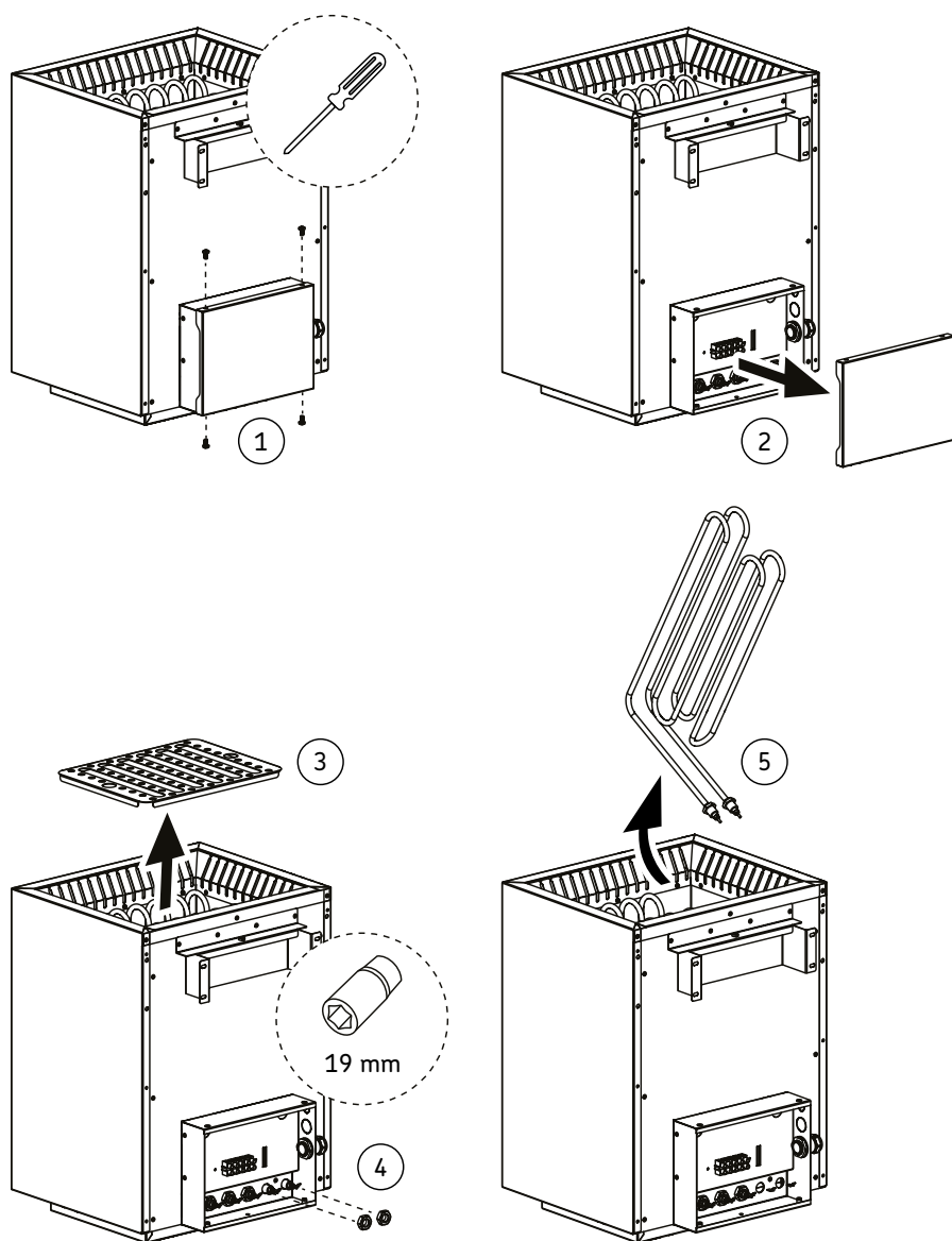
Obrázek 14 Výměna topných těles
