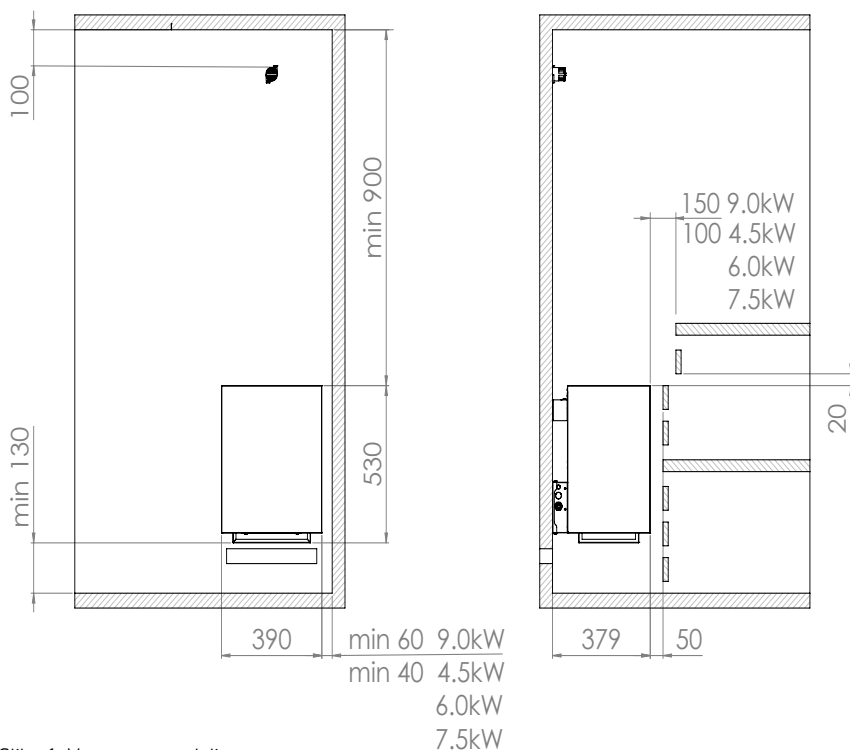
Slika 1. Varnostne razdalje
