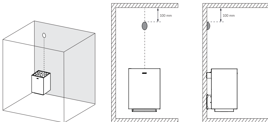
Figura 3. Instalación del sensor térmico en la pared
