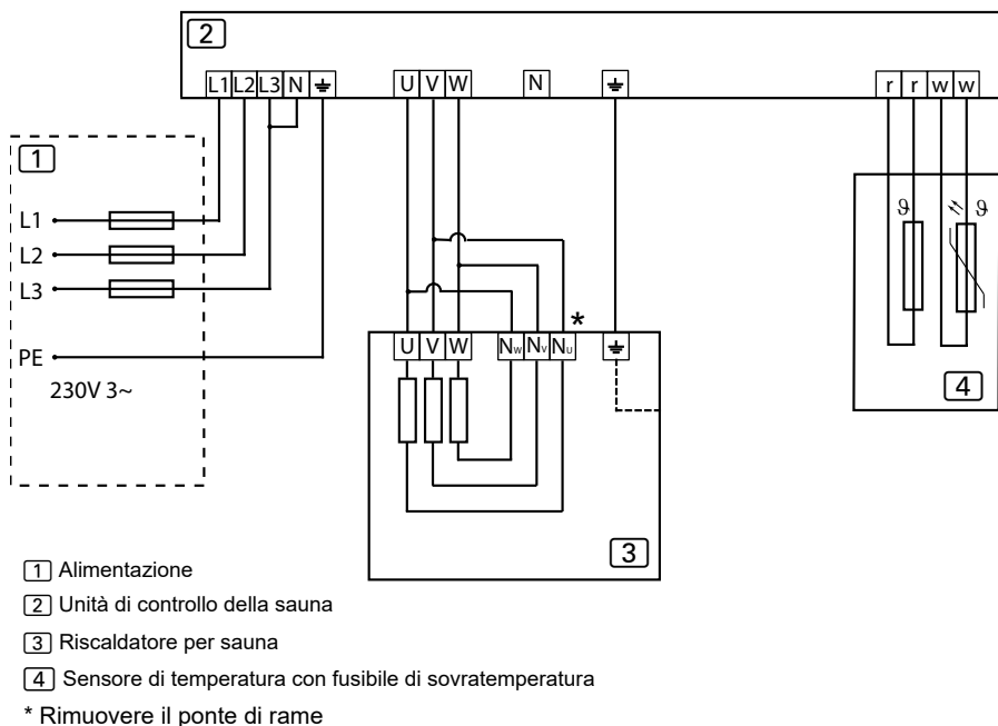
Figura 11. Schema elettrico 230V 3~
