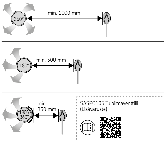
Kuva 13. Tuloilmaventtiilin vähimmäisetäisyys lämpötila-anturiin
