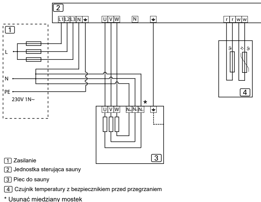
Rysunek 10. Schemat połączeń 230V 1N~
