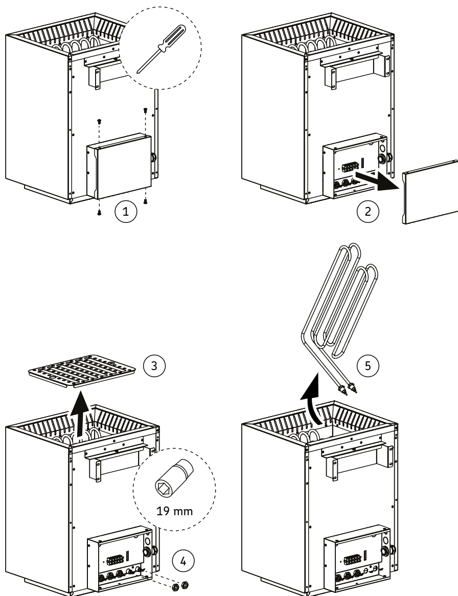
Slika 14. Menjava grelnih elementov
