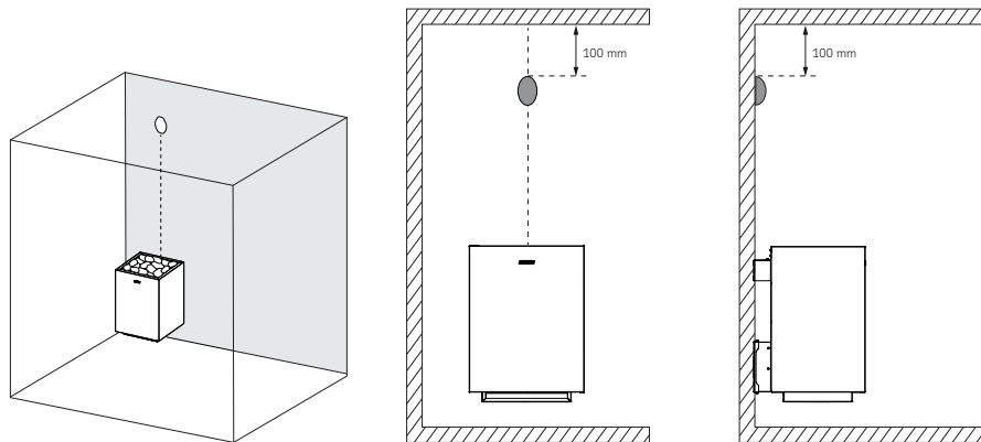
3. attēls. Siltuma sensora uzstādīšana pie sienas
