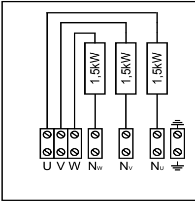
Kuva 5. Kytentäkaavio HLW45E
