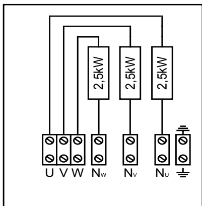
Obrázek 7. Schéma zapojení HLW75E
