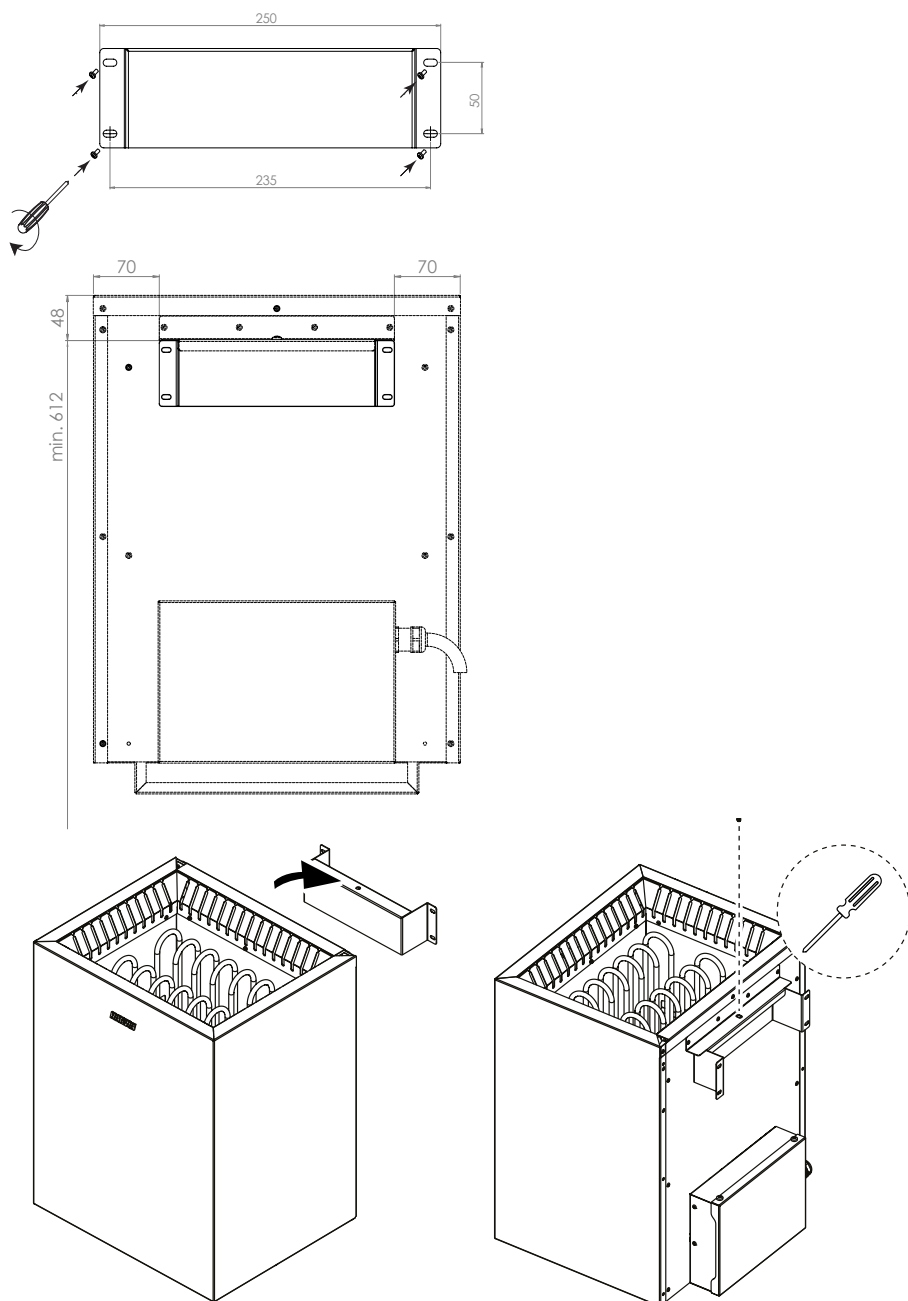
Figura 2. Installazione della stufa per sauna
