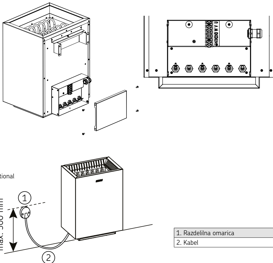
Slika 4. Električni priključki
