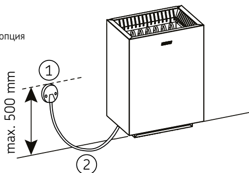
Рисунок 4. Электрические соединения
