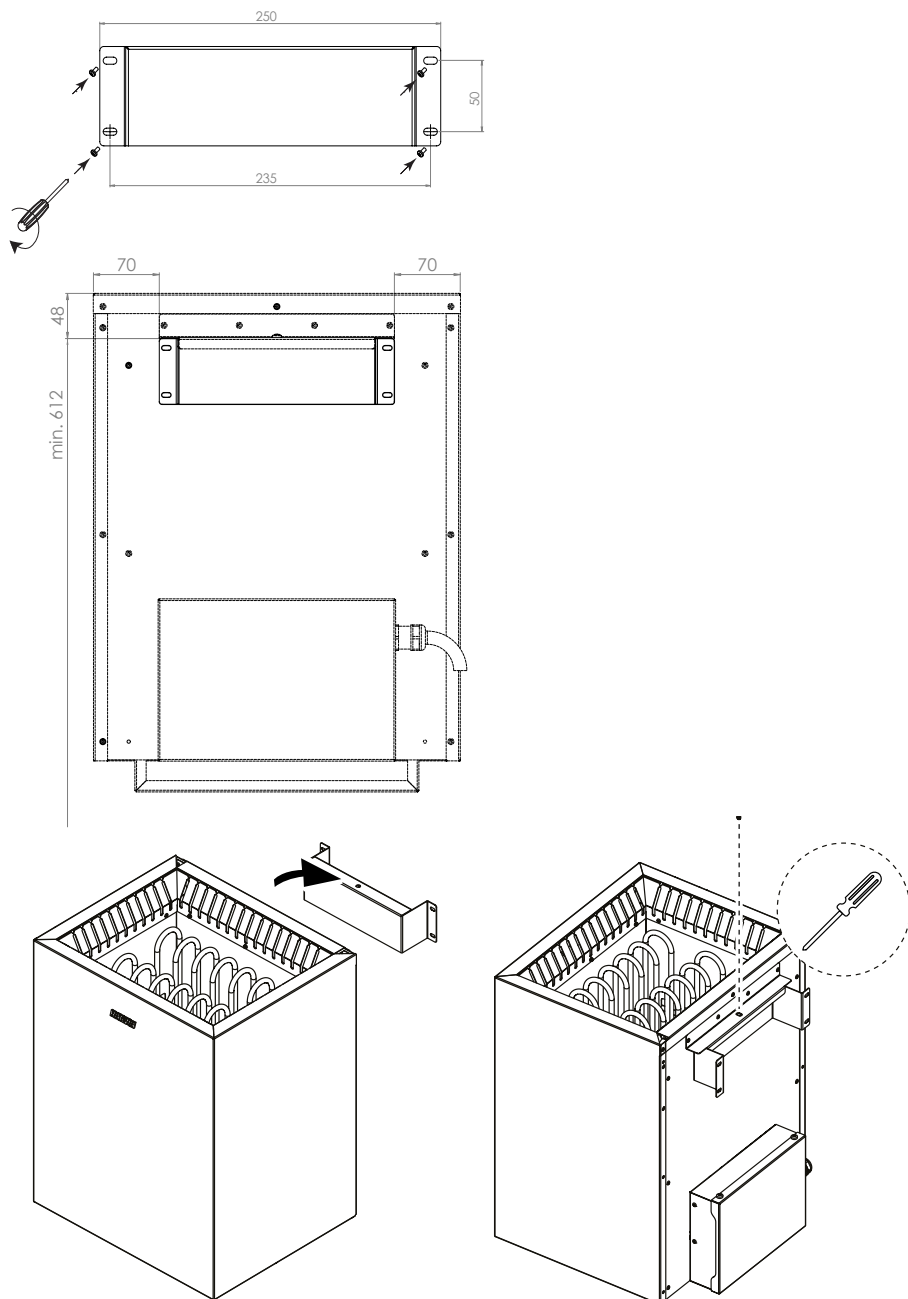
Figuur 2. Installatie saunakachel
