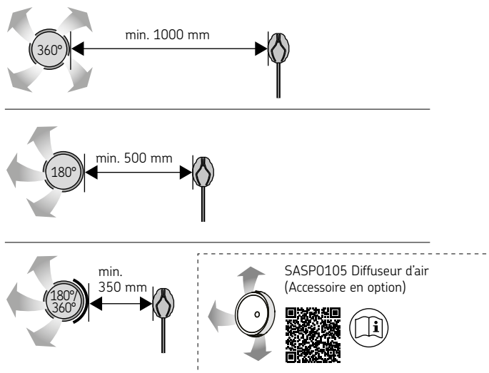
Figure 13. Distance minimale entre la bouche d'air et le capteur
