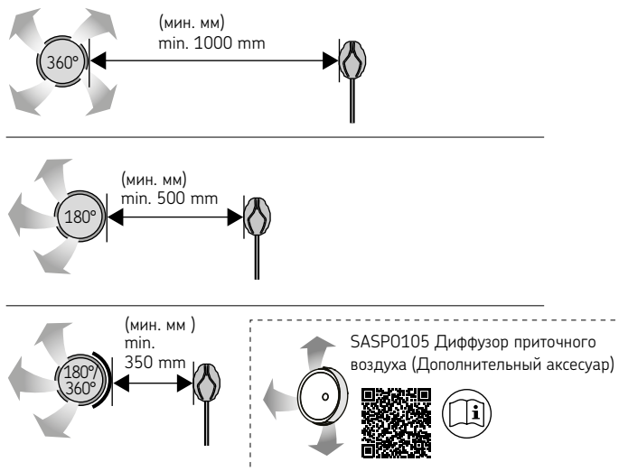
Рисунок 13. Минимальное расстояние от температурного датчика до вентиляционной отдушины.
