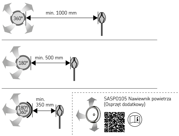
Rysunek 13. Minimalna odległość otworu wentylacyjnego od czujnika.
