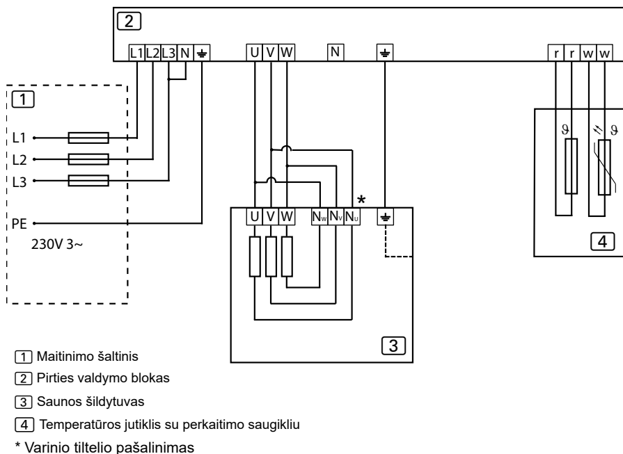
11 pav. Laidų prijungimo schema 230V 3~
