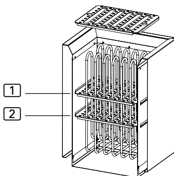
Figure 12. Placement des pierres de poêle
