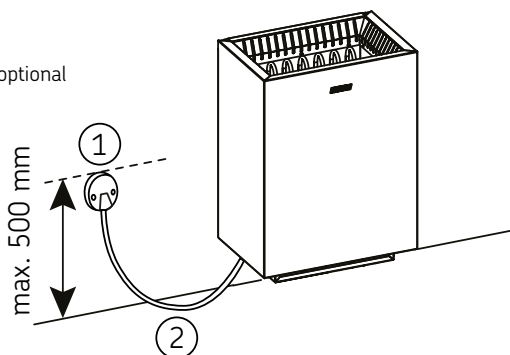
Rysunek 4. Połączenia elektryczne
