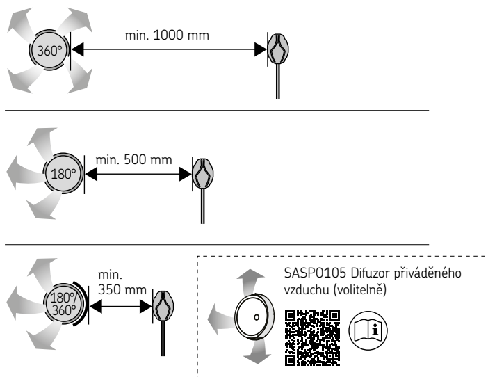
Obrázek 13. Minimální vzdálenost od větracího otvoru přívodu vzduchu k teplotnímu senzor
