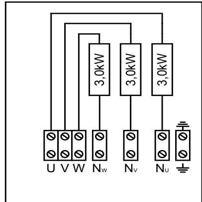
Bild 8. Kopplingsschema HLW90E
