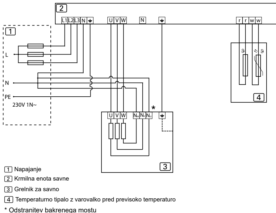
Slika 10. Shema ožičenja 230V 1N~
