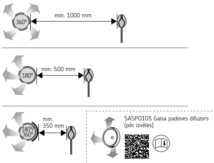
13. attēls. Minimālais attālums no gaisa padeves lūkas līdz temperatūras sensoram
