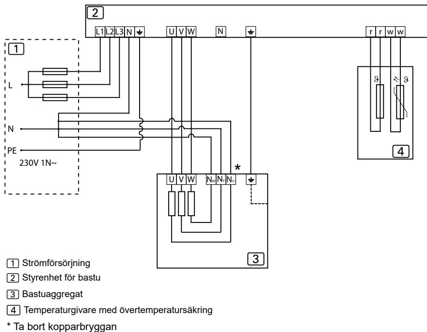
Bild 10. Kopplingsschema 230V 1N~
