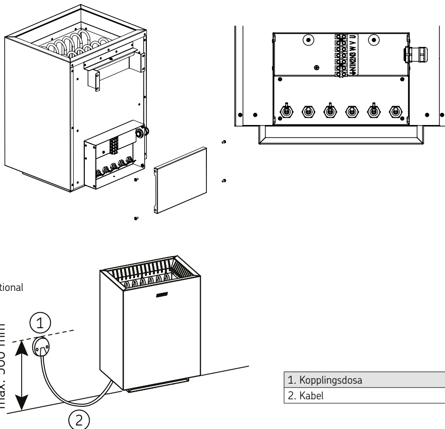
Bild 4. Elinstallation
