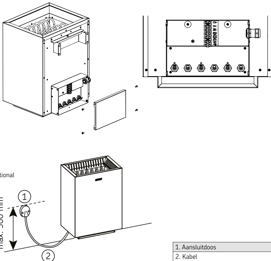
Figuur 4. Elektrische aansluitingen
