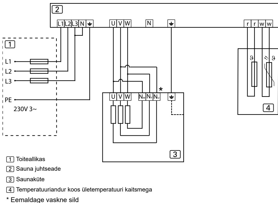
Joonis 11. Elektriskeem 230V 3~
