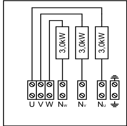
Kuva 8. Kytentäkaavio HLW90E
