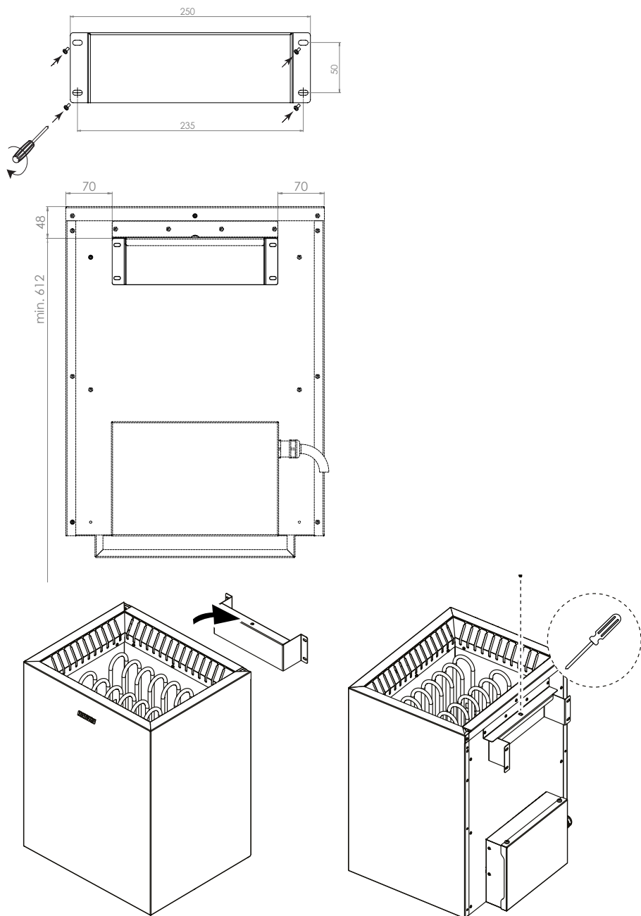
Figure 2. Installation du poêle pour sauna
