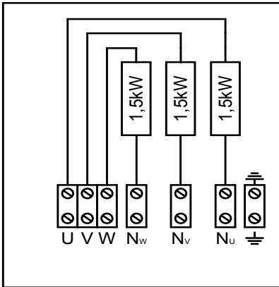
Bild 5. Kopplingsschema HLW45E
