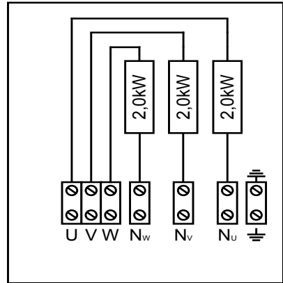
Bild 6. Kopplingsschema HLW60E
