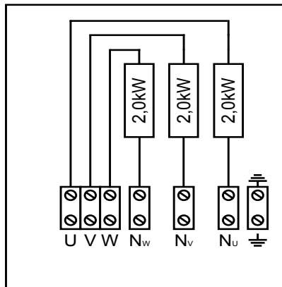
Figuur 6. Aansluitschema HLW60E
