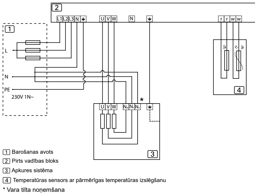
10. attēls. Savienojuma shēma 230V 1N~
