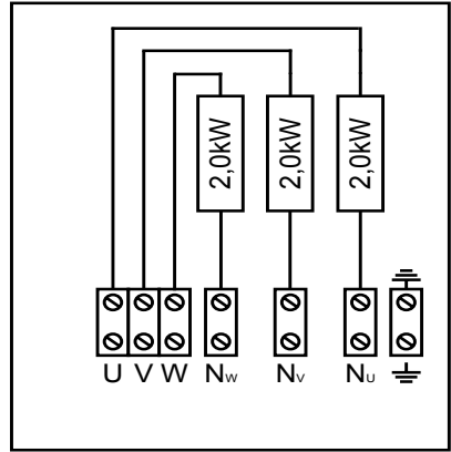
Kuva 6. Kytentäkaavio HLW60E
