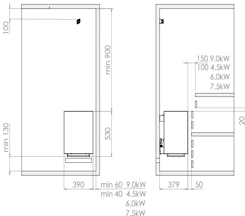
Bild 1. Säkerhetsavstånd
