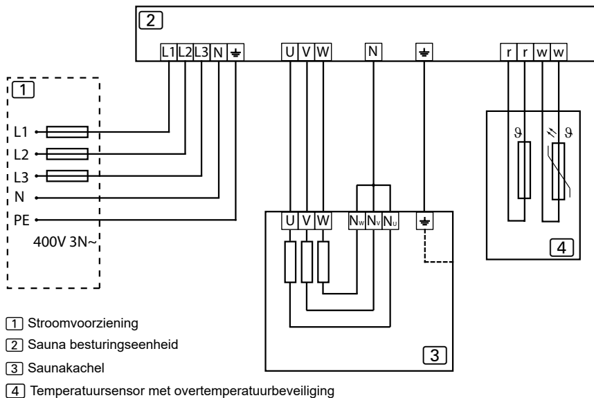
Figuur 9. Aansluitschema 400V 3N~
