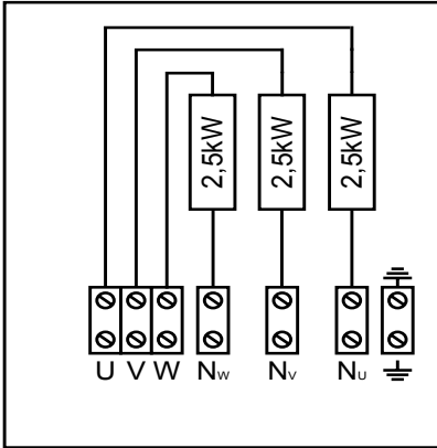
Kuva 7. Kytentäkaavio HLW75E
