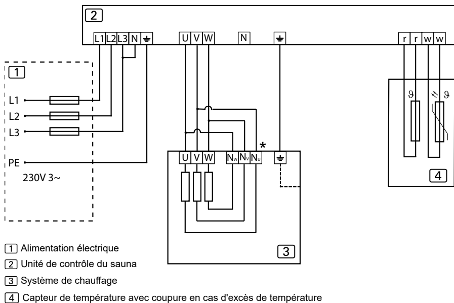
Figure 11. Schéma de câblage 230V 3~
