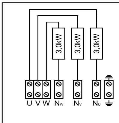
Rysunek 8. Schemat połączeń HLW90E
