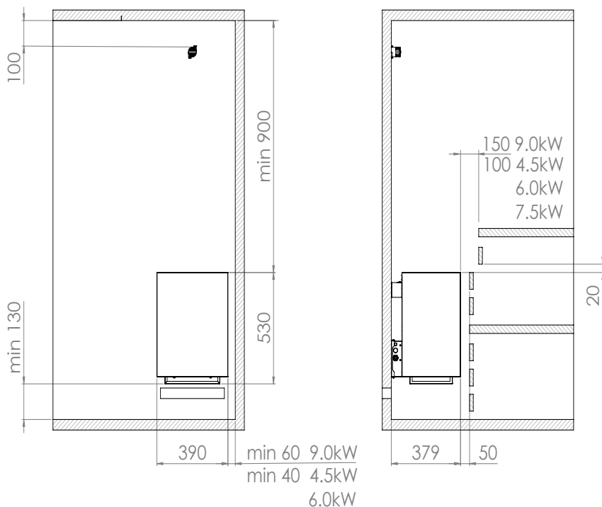
Joonis 1. Ohutuskaugused
