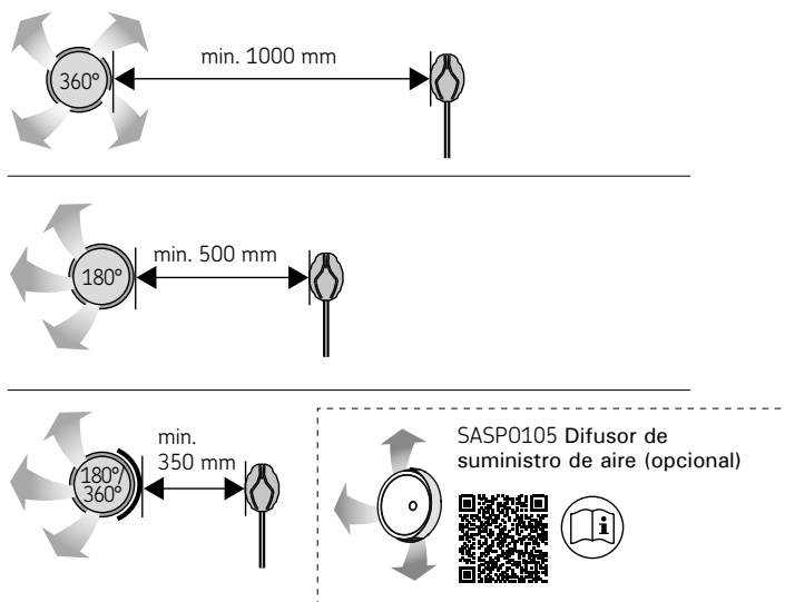
Figura 13. Distancia mínima entre la salida de suministro de aire y el sensor de temperatura
