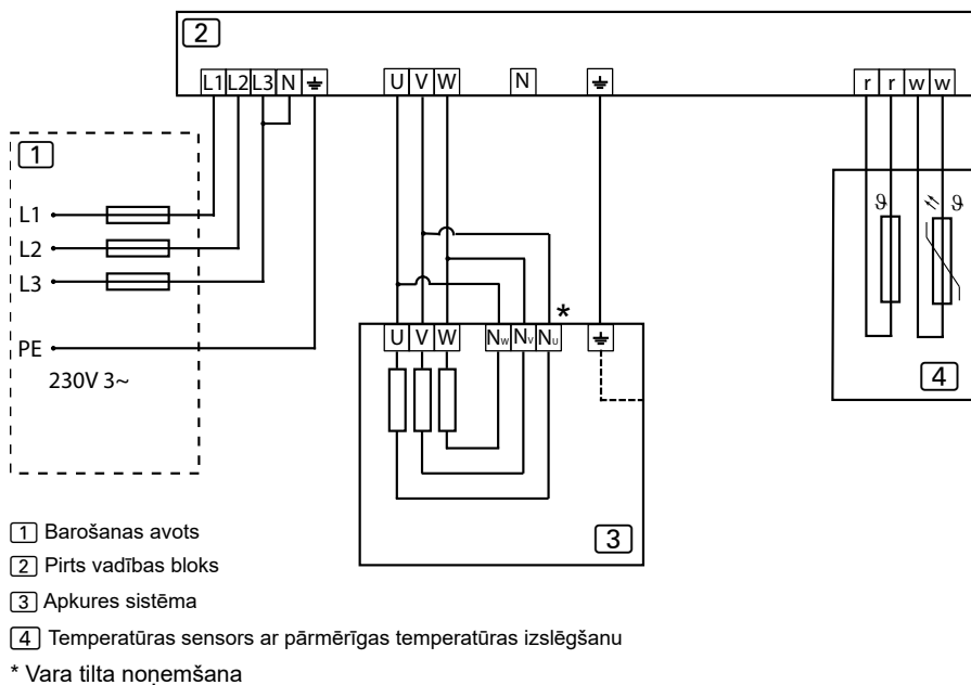
11. attēls. Savienojuma shēma 230V 3~
