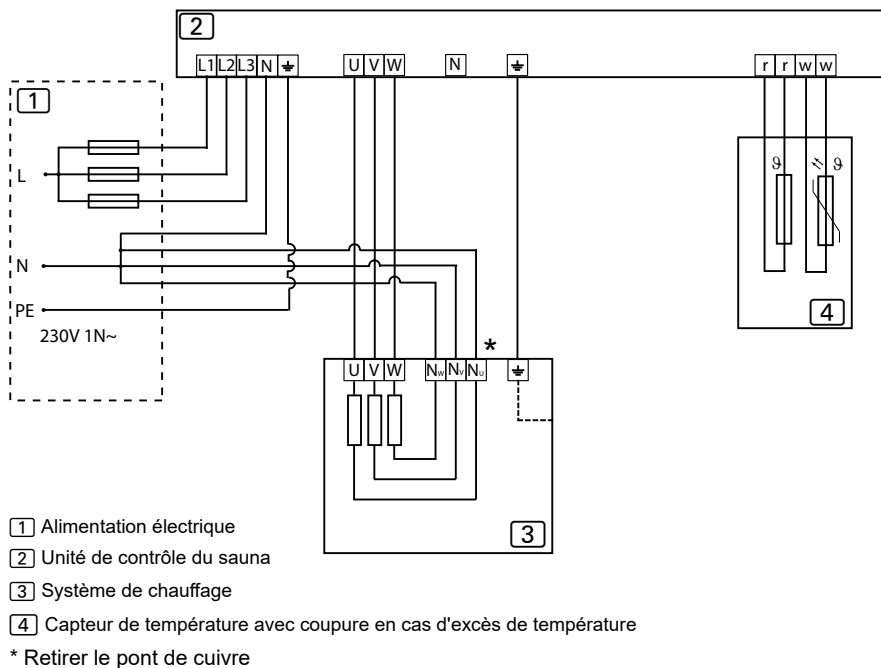
Figure 10. Schéma de câblage 230V 1N~
