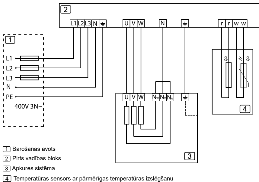
9. attēls. Savienojuma shēma 400V 3N~
