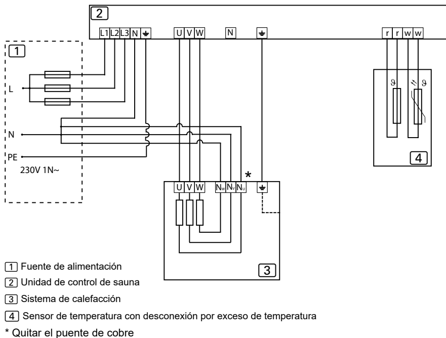
Figura 10. Diagrama de conexiones 230V 1N~
