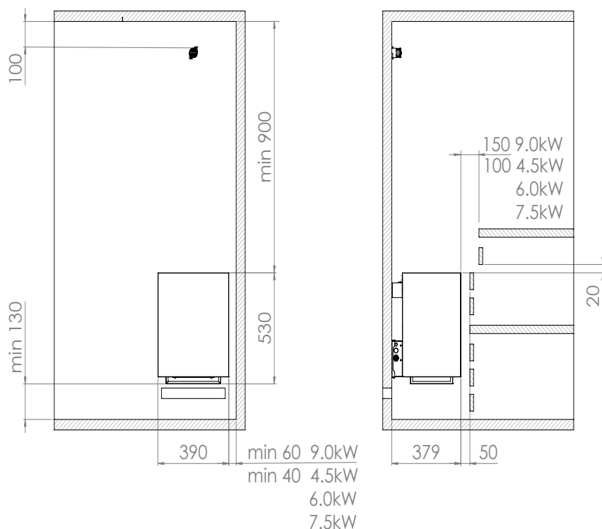
Obrázek 1 Bezpečnostní vzdálenosti
