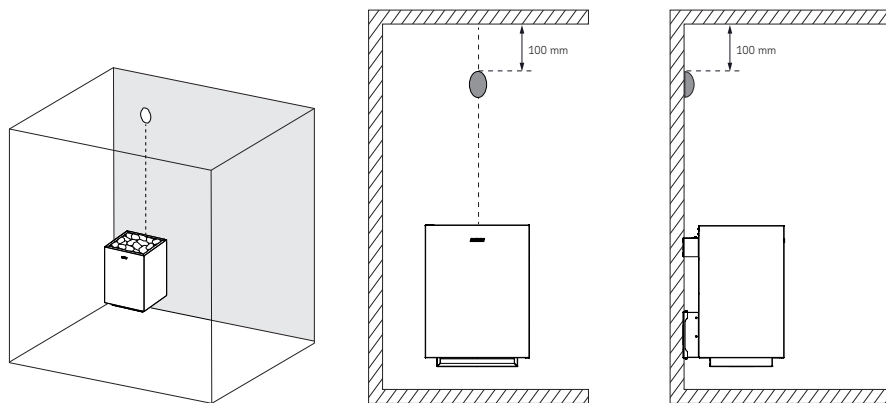
Slika 3. Namestitev toplotnega senzorja na steno
