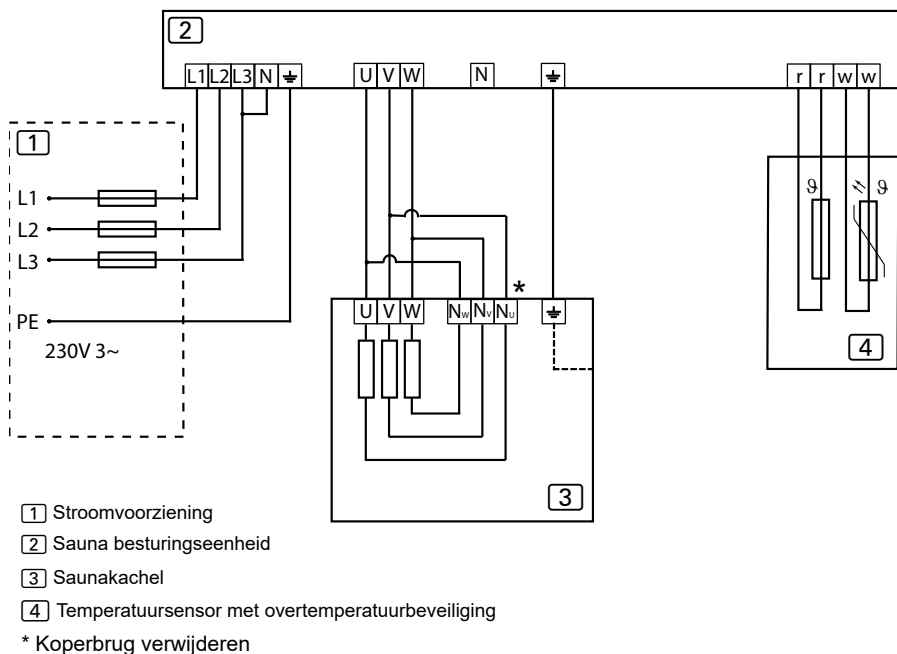
Figuur 11. Aansluitschema 230V 3~
