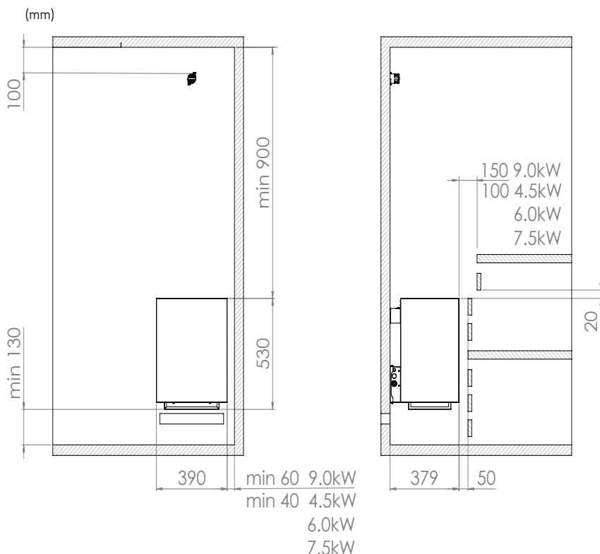
Figuur 1. Veiligheidsafstanden
