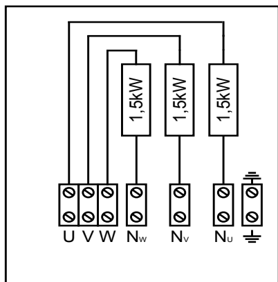
Slika 5. Shema ožičenja HLW45E
