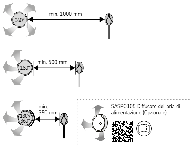
Figura 13. Distanza minima tra lo sfizio dell'aria di alimentazione e il sensore di temperatura.
