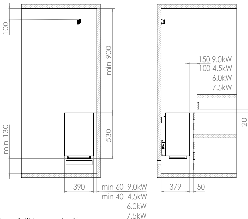
Figure 1. Distances de sécurité
