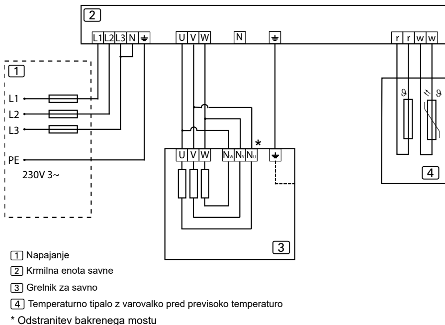
Slika 11. Shema ožičenja 230V 3~
