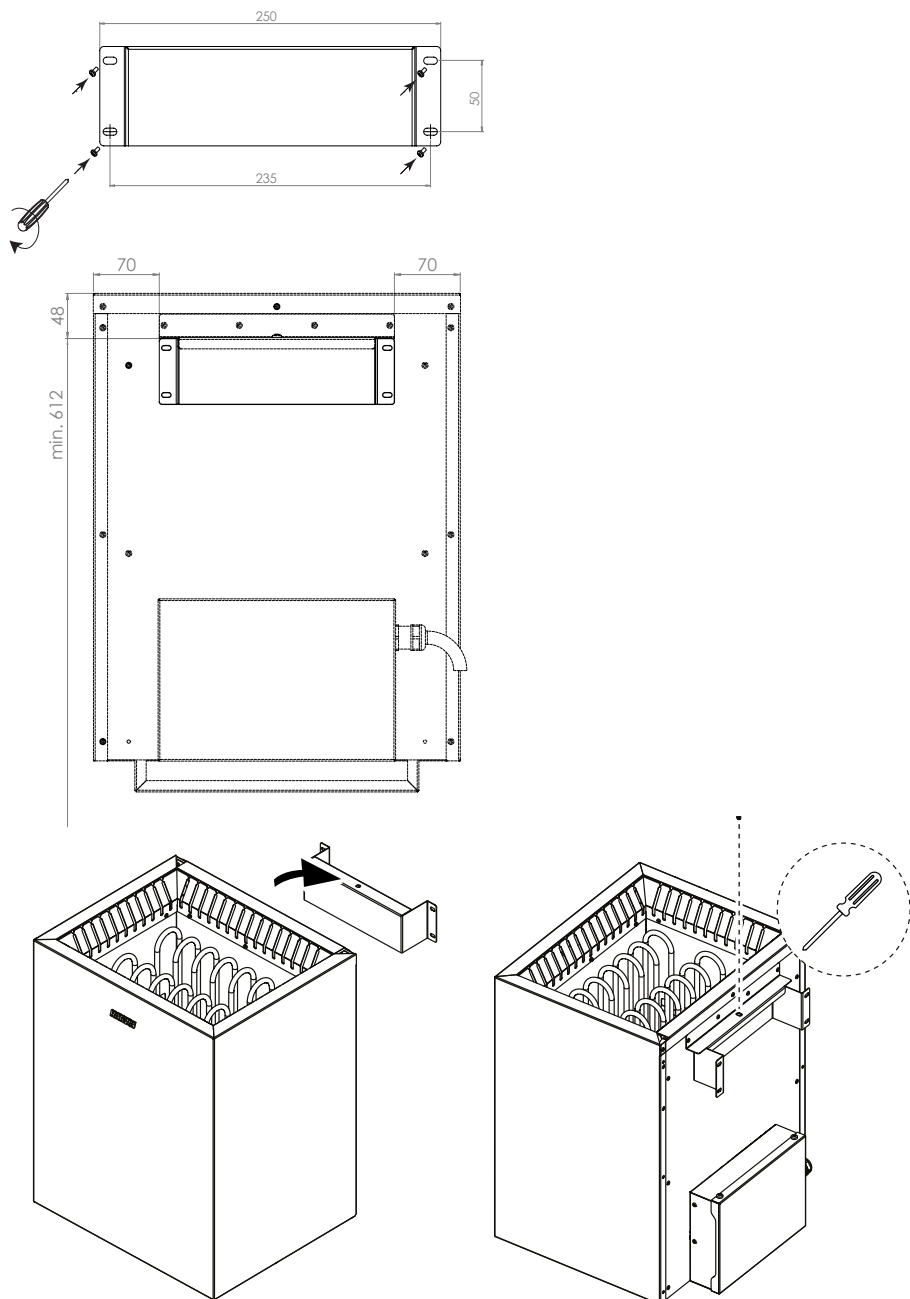
Slika 2. Namestitev grelca za savno
