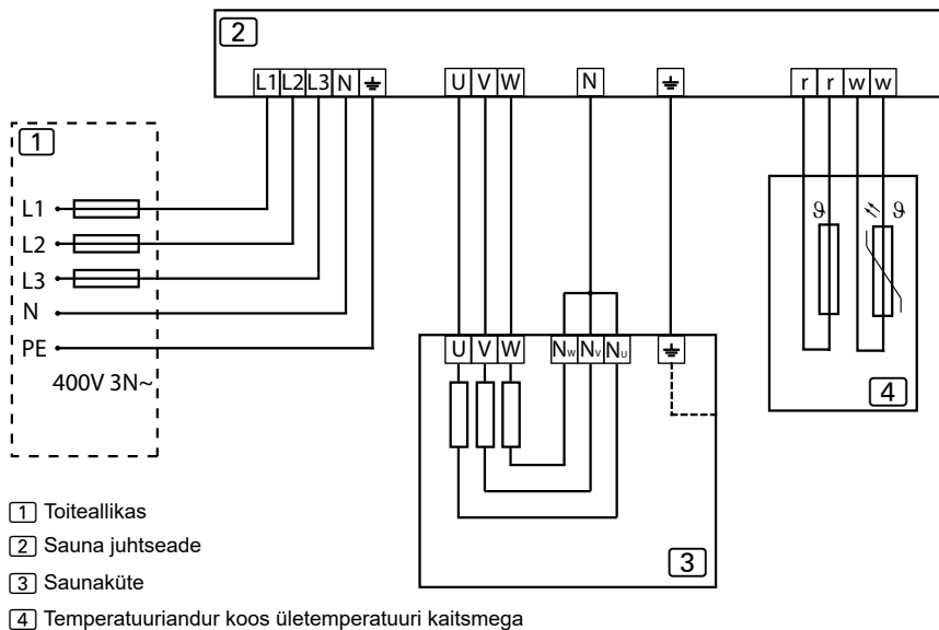
Joonis 9. Elektriskeem 400V 3N~
