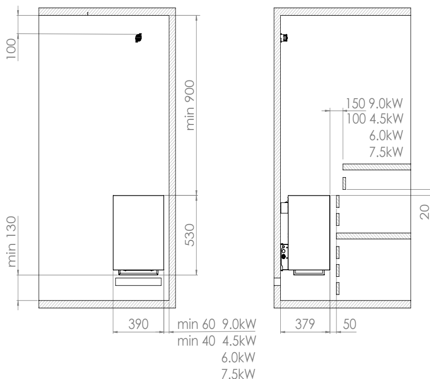
Figura 1. Distanza di sicurezza
