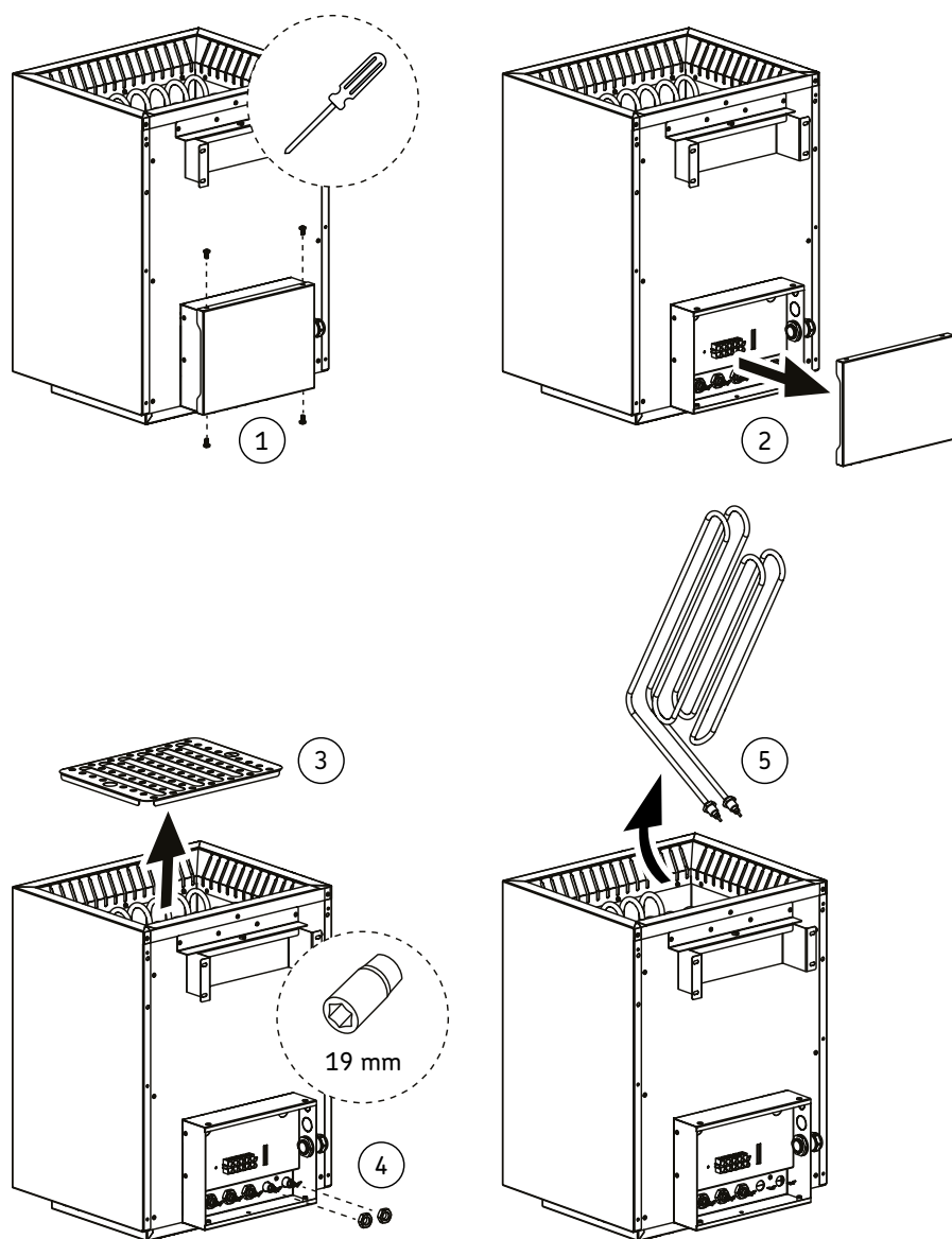
Joonis 14. Kütteelementide vahetamine
