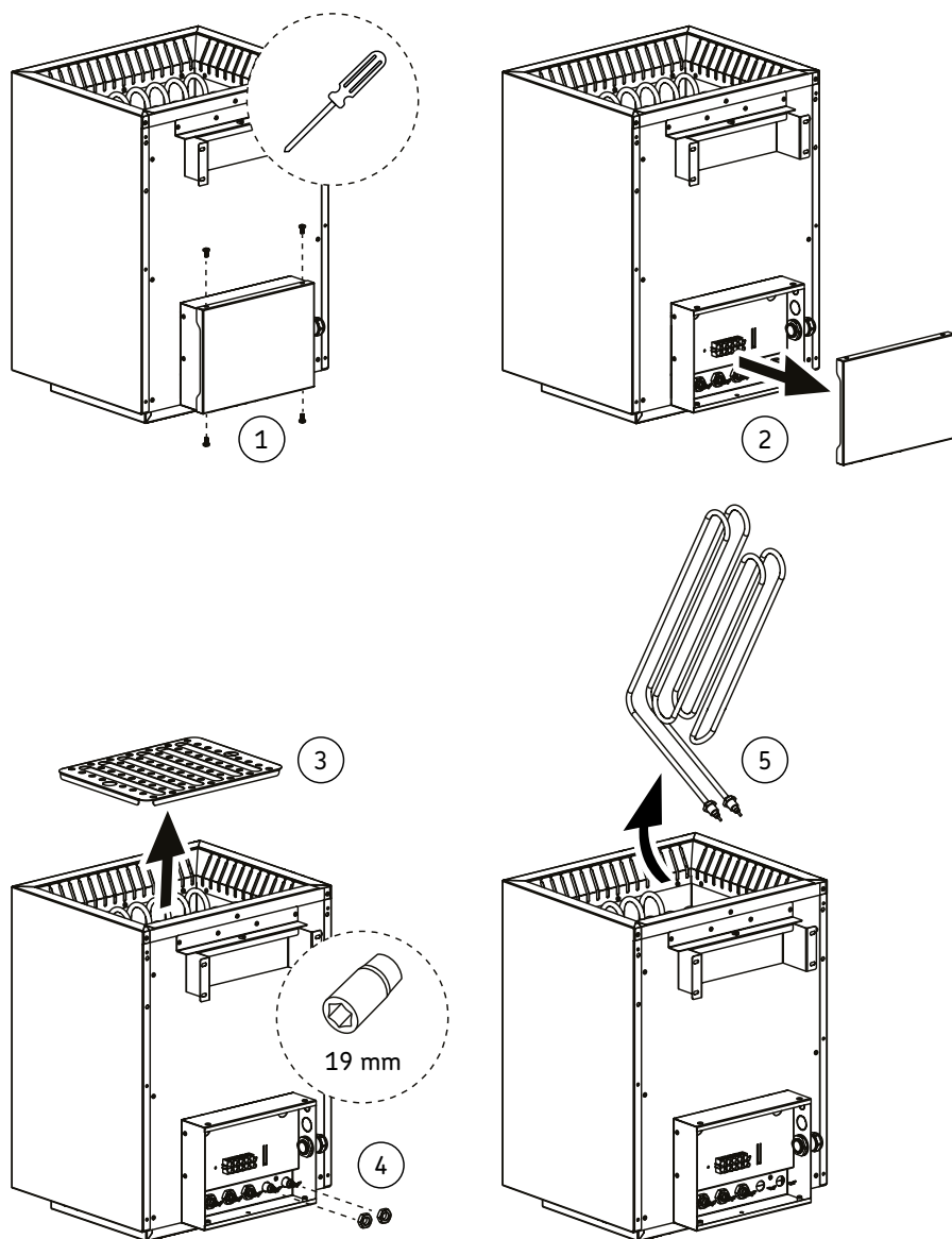
Рисунок 14. Замена нагревательных элементов
