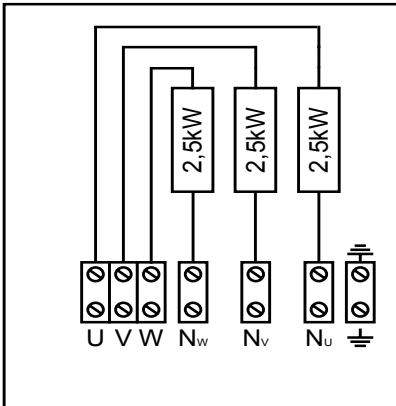
Bild 7. Kopplingsschema HLW75E
