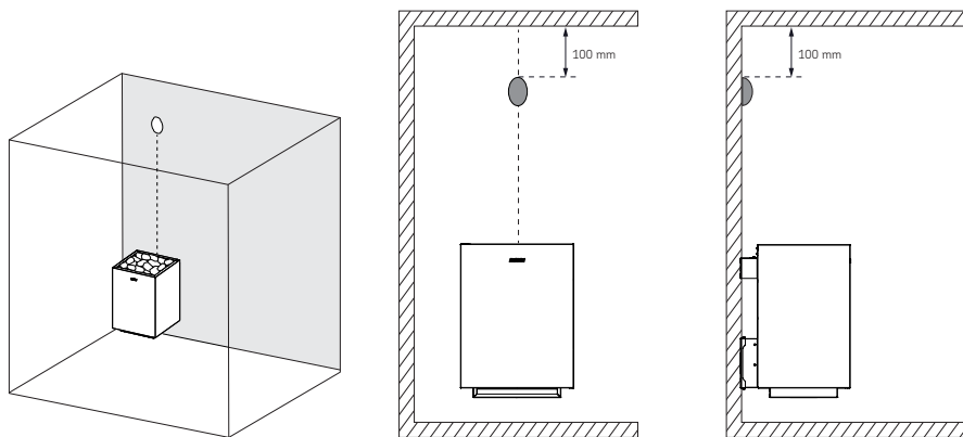
Rysunek 3. Montaż czujnika ciepła na ścianie
