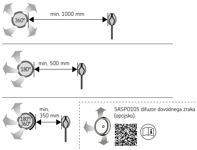
Slika 13. Najmanjša razdalja od zračnika za dovod zraka do senzorja za temperaturo.
