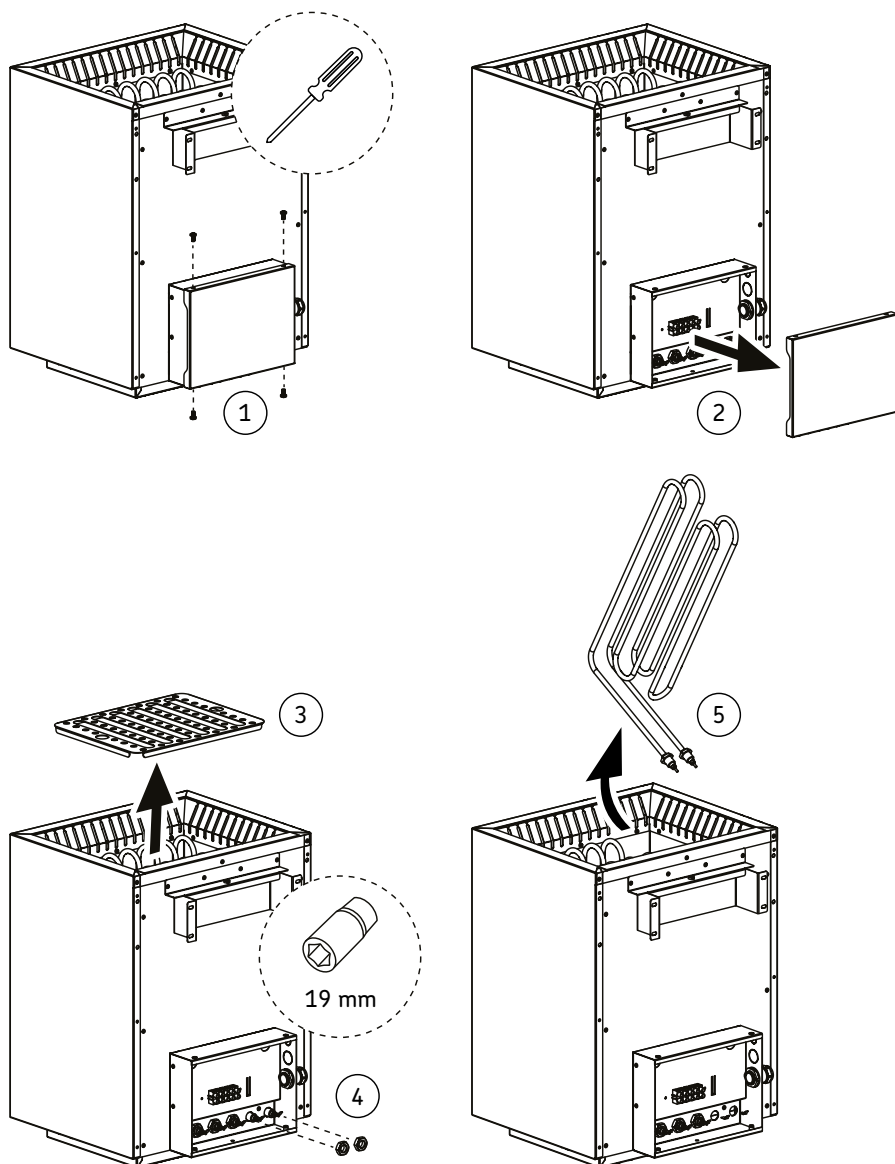
14. attēls. Sildelementu maiņa
