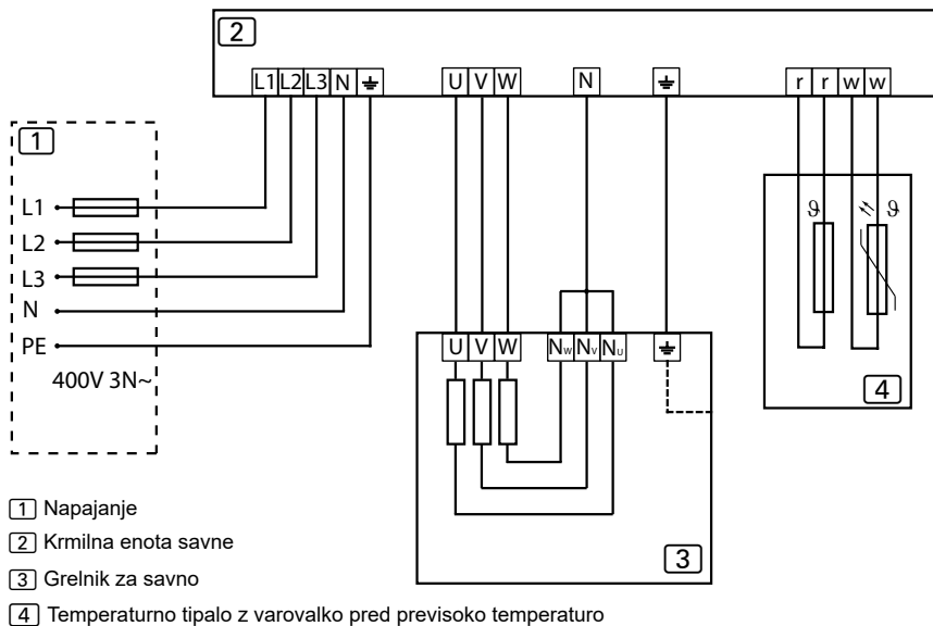
Slika 9. Shema ožičenja 400V 3N~
