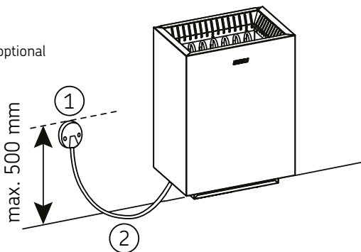
Kuva 4. Sähkökytkennät
