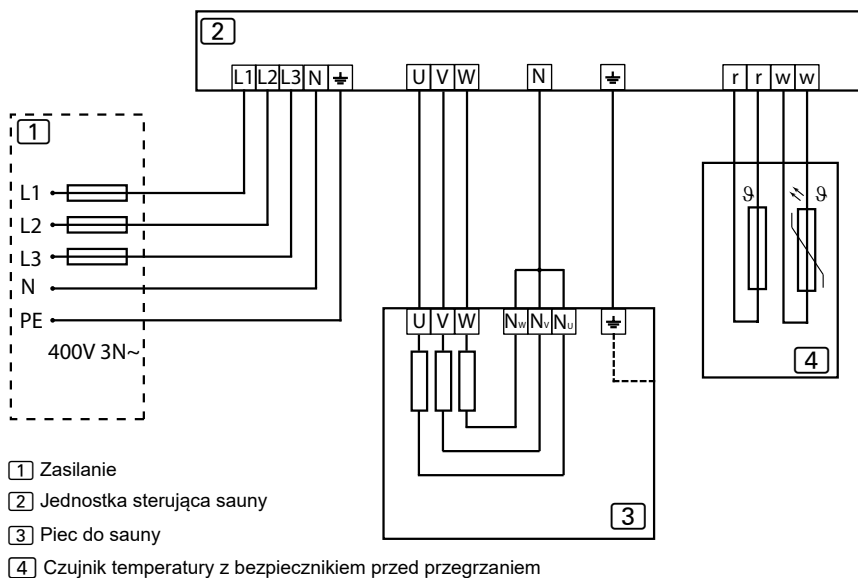
Rysunek 9. Schemat połączeń 400V 3N~
