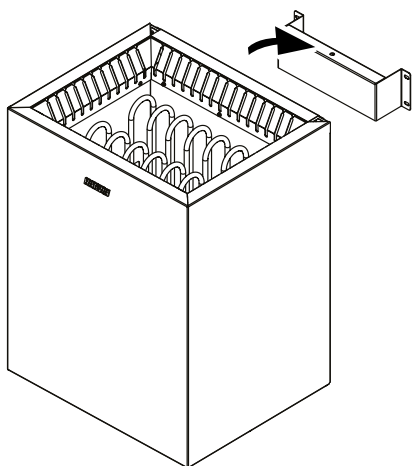
2. attēls. Pirts sildītāja uzstādīšana
