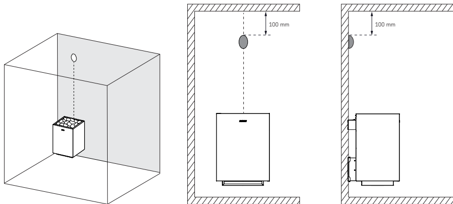
3 pav. Šilumos jutiklio montavimas ant sienos
