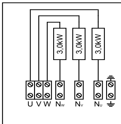
Figuur 8. Aansluitschema HLW90E
