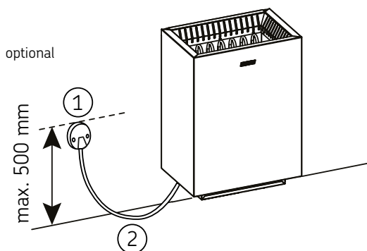
Joonis 4. Elektriühendused
