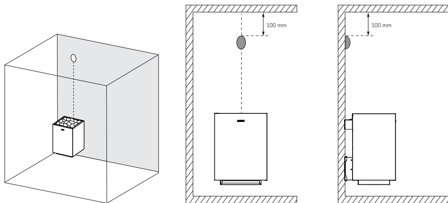
Рисунок 3. Установка термостата на стене
