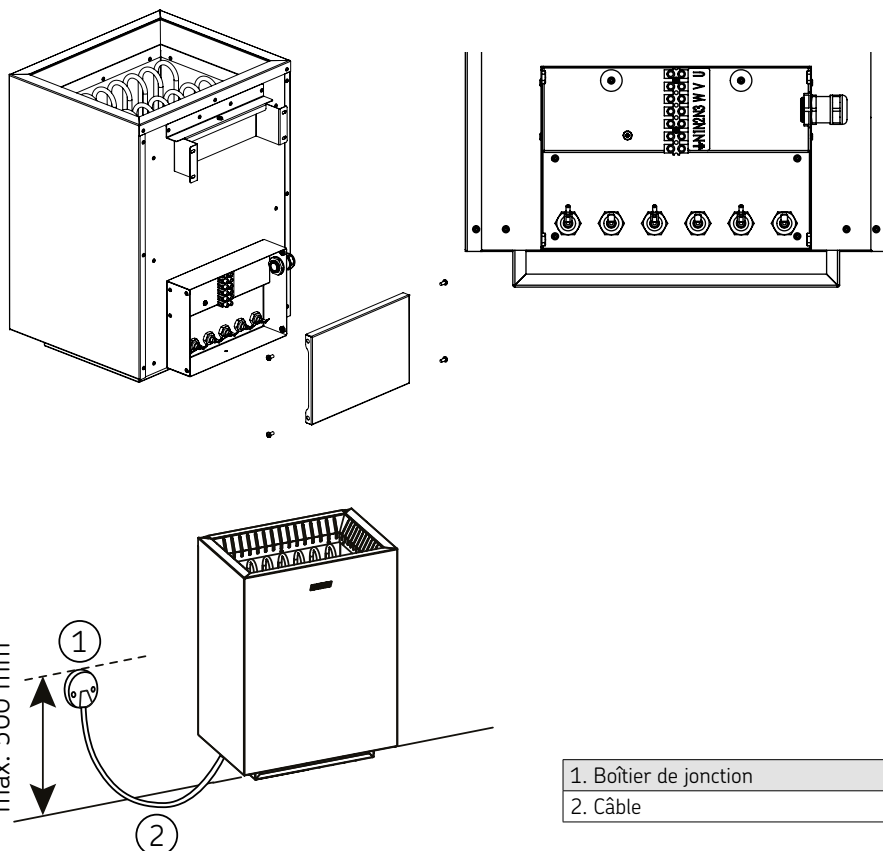
Figure 4. Raccordements électriques
