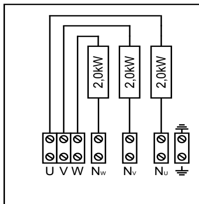
6. attēls. Elektroinstalācijas shēma HLW60E
