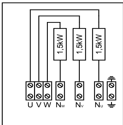
Figure 5. Schéma de câblage HLW45E
