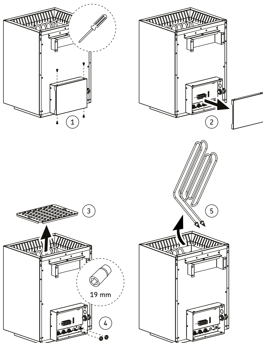
Figura 14. Sostituzione delle resistenze
