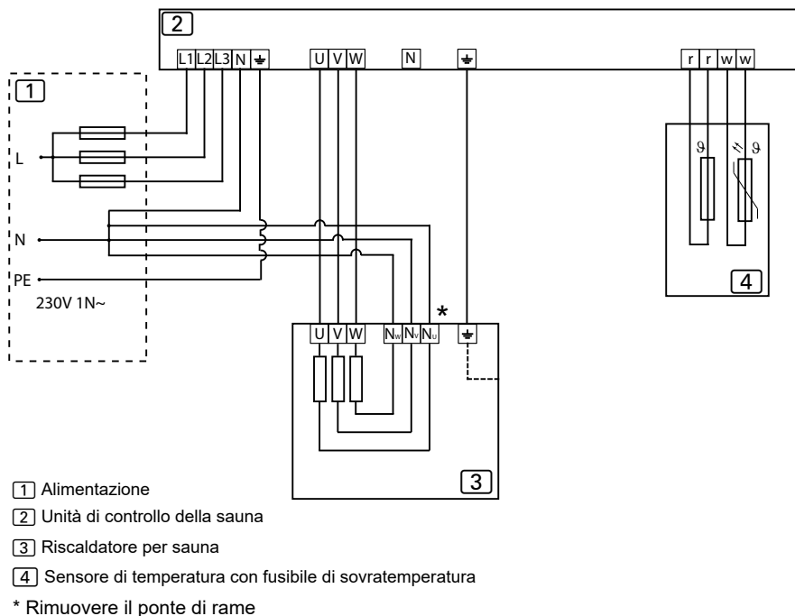
Figura 10. Schema elettrico 230V 1N~
