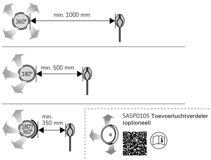
Figuur 13. Minimale afstand van de luchttoevoerklap tot de temperatuursensor.
