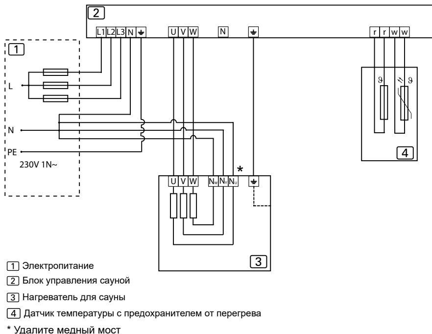
Рисунок 10. Электрическая схема 230V 1N~
