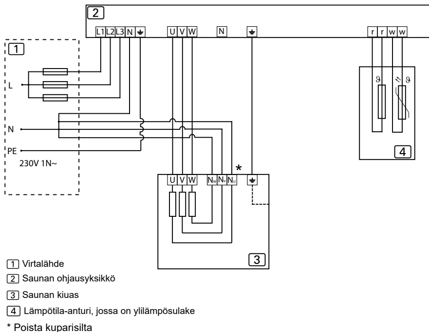
Kuva 10. Kytentäkaavio 230V 1N~
