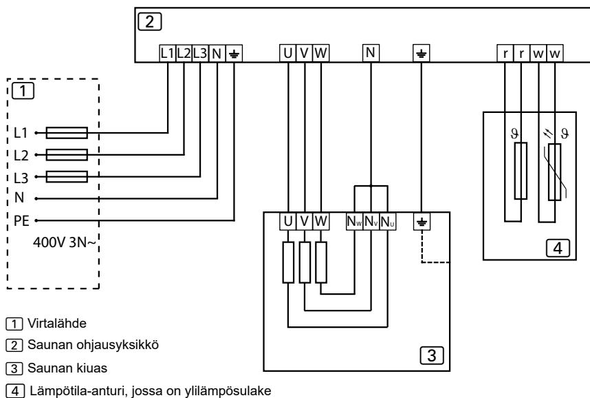
Kuva 9. Kytentäkaavio 400V 3N~
