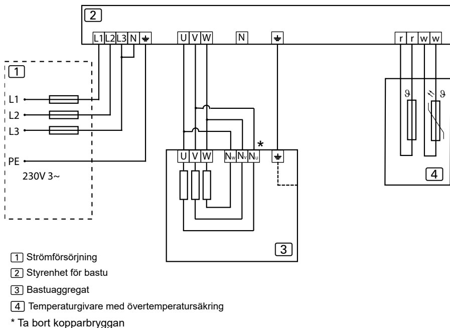
Bild 11. Kopplingsschema 230V 3~
