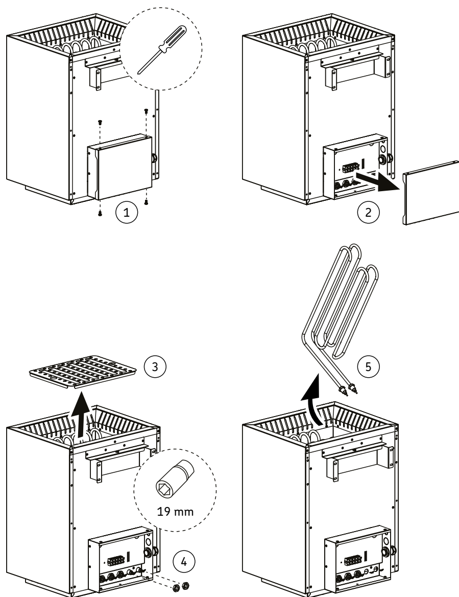
Rysunek 14. Wymiana elementów grzejnych
