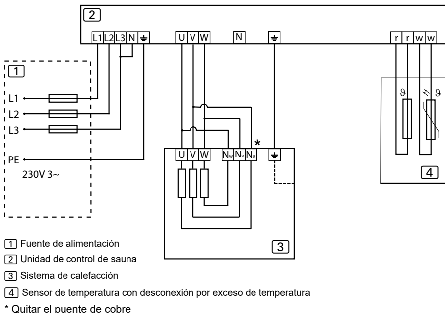
Figura 11. Diagrama de conexiones 230V 3~
