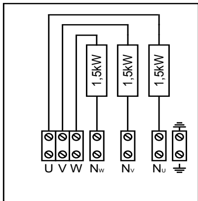
Figuur 5. Aansluitschema HLW45E
