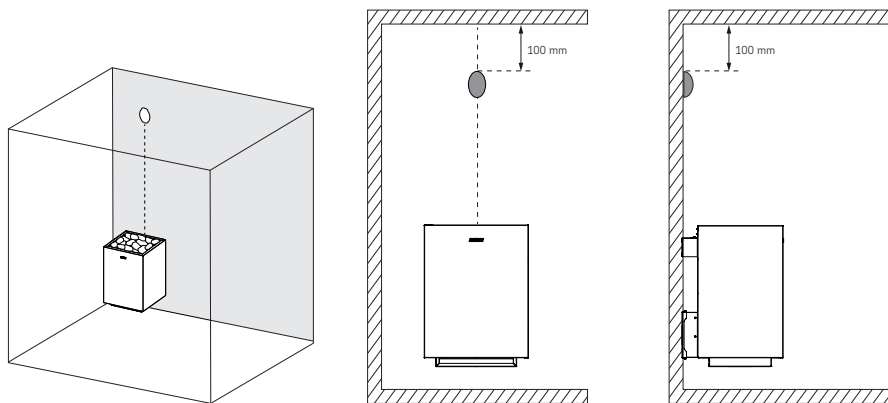
Bild 3. Installera värmegivaren på väggen
