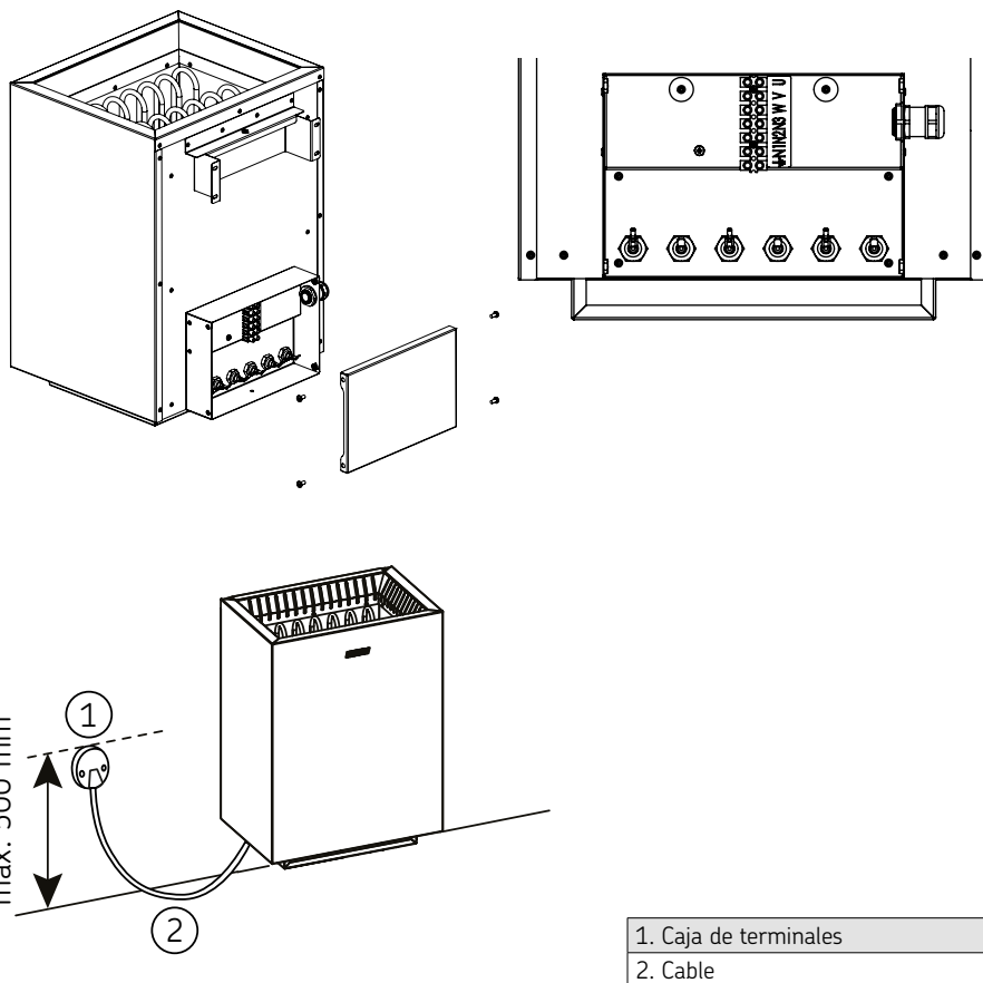
Figura 4. Conexiones eléctricas
