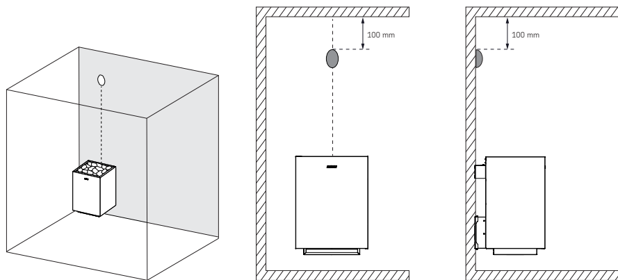
Joonis 3. Soojusanduri paigaldamine seinale
