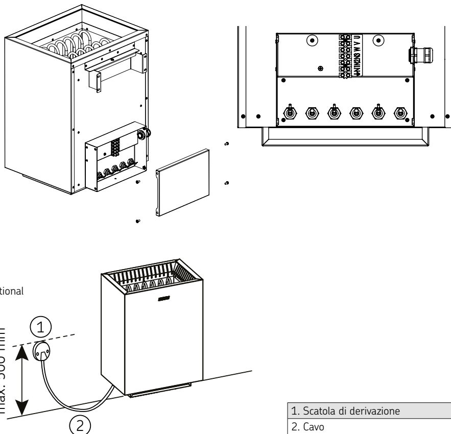
Figura 4. Collegamenti elettrici
