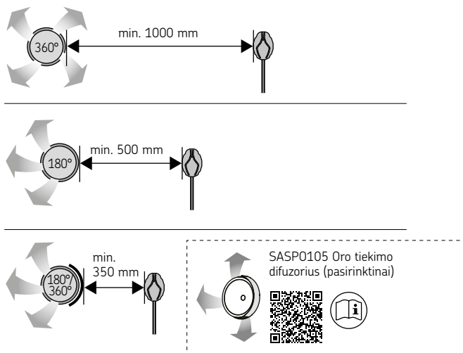
13 pav. Mažiausias atstumas nuo tiekiamo oro ventiliacijos angos iki temperatūros jutiklio
