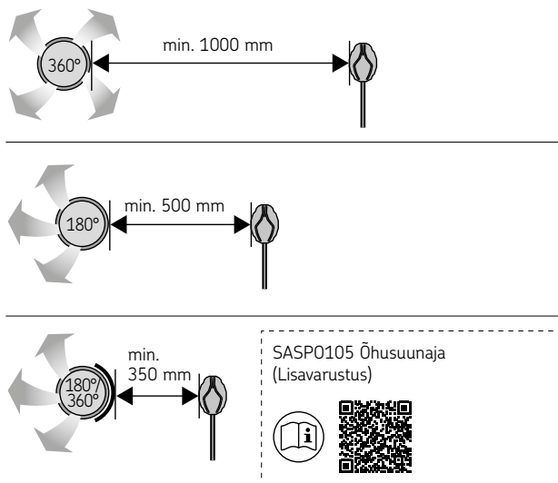
Joonis 13. Ventilatsiooniava minimaalne kaugus andurist.
