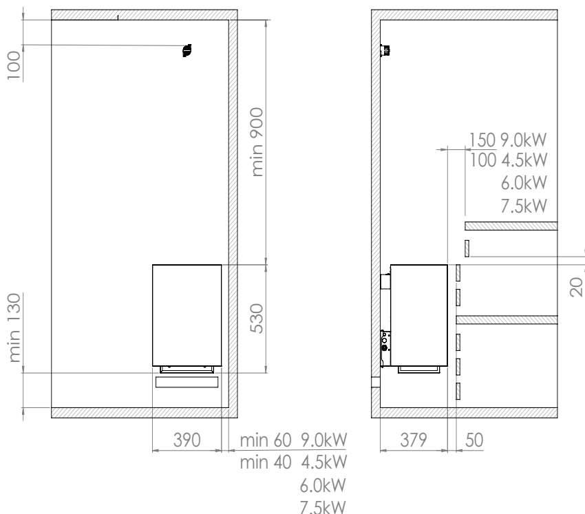
Rysunek 1. Odległości bezpieczeństwa
