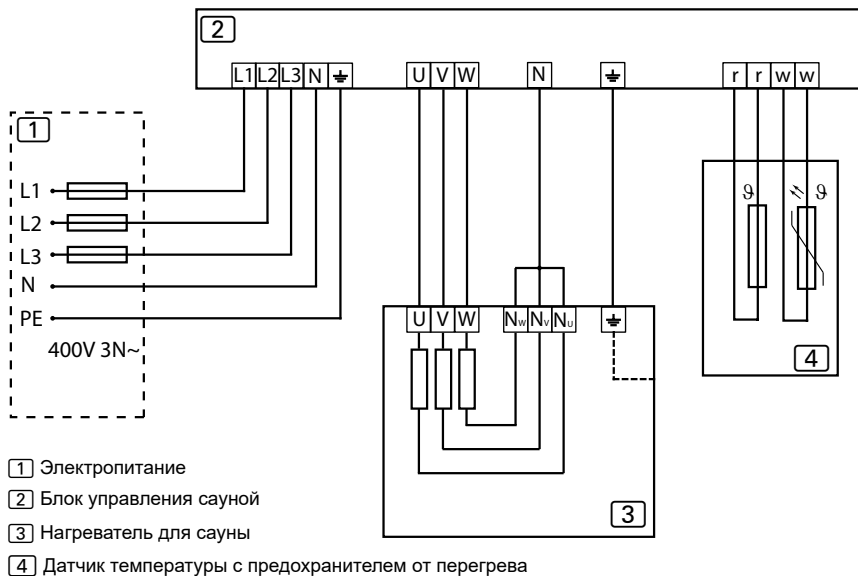
Рисунок 9. Электрическая схема 400V 3N~
