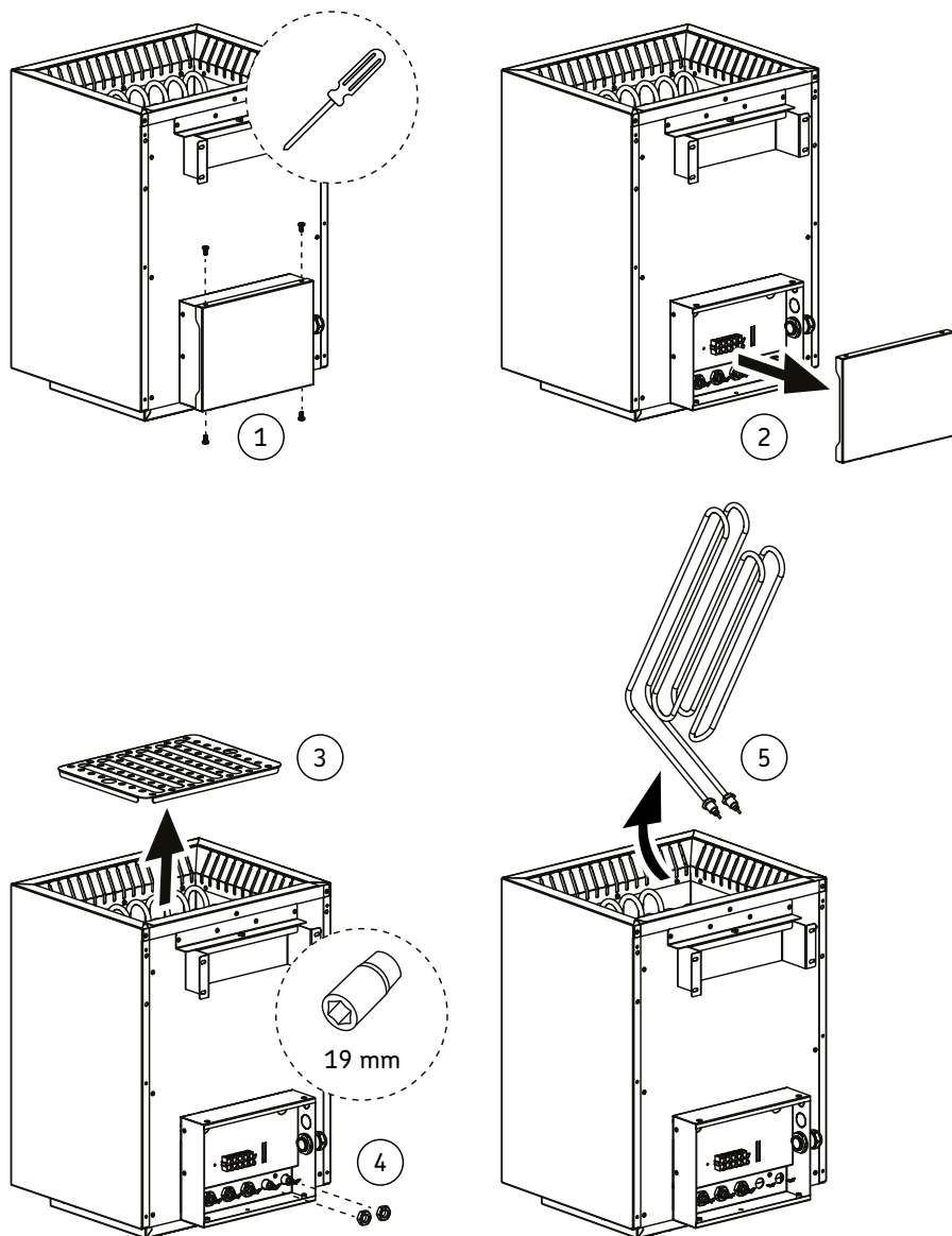
Figure 14. Remplacement des résistances
