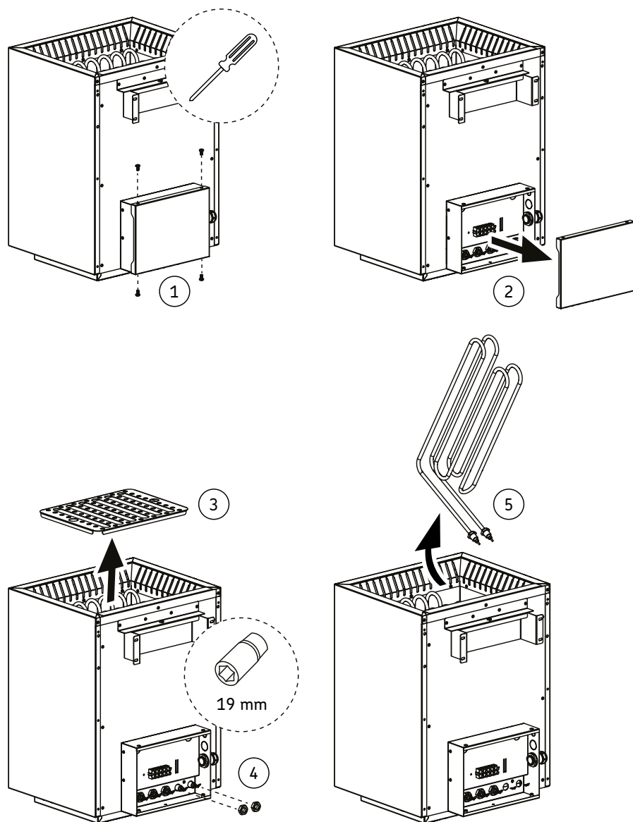
Bild 14. Byta värmeelement
