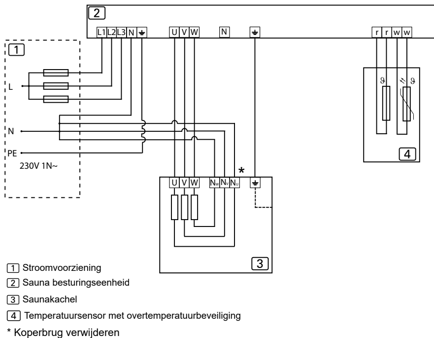
Figuur 10. Aansluitschema 230V 1N~
